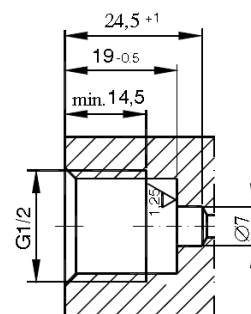
Рисунок Д.4б Гнездо для присоединения типа «G \frac{1}{2} »
