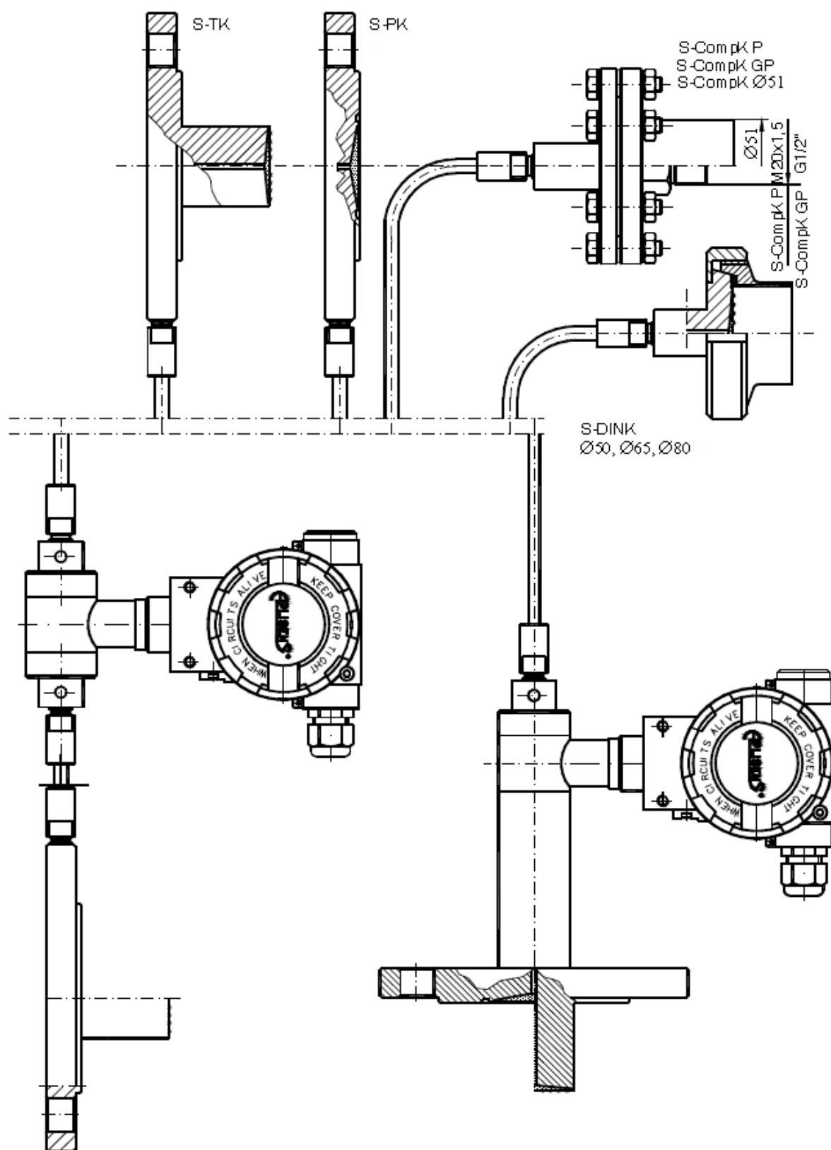
Рисунок Б.3 - Внешний вид, установочные и присоединительные размеры преобразователей APR-2200/ALW/Exd
