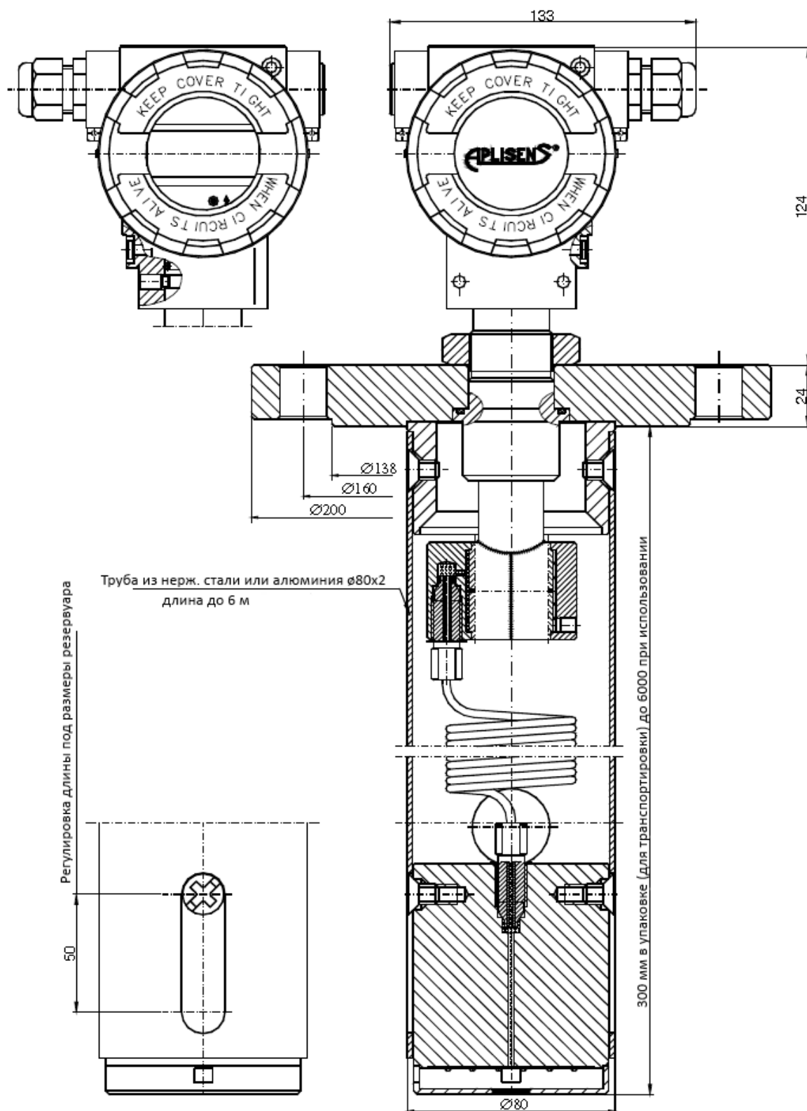
Рисунок Б.4 - Внешний вид, установочные и присоединительные размеры преобразователей APR-2000Y/ALW/Exd
