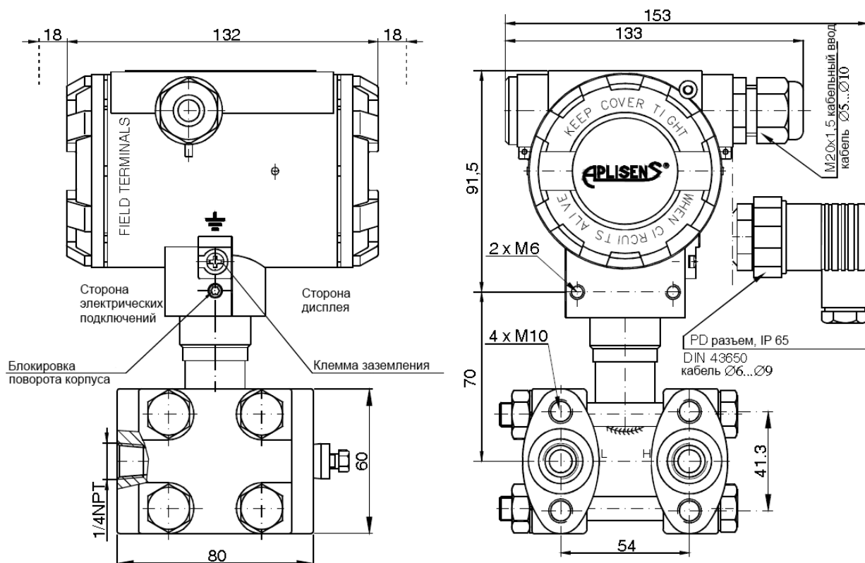
Рисунок Б.2- Внешний вид, установочные и присоединительные размеры преобразователей APR-2000/ALW/Exd с присоединением типа С
