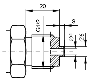
Рисунок Д.4а Присоединение типа «G \frac{1}{2} », с резьбой G \frac{1}{2} ''
