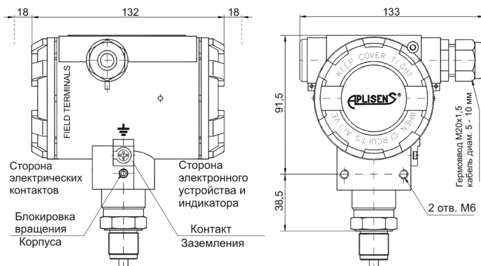
Рисунок Б.1- Внешний вид, установочные и присоединительные размеры преобразователей APC-2000/ALW/Exd
