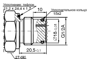
Рисунок Д.5а Присоединение типа «CG \frac{1}{2} », с резьбой G \frac{1}{2} ''
